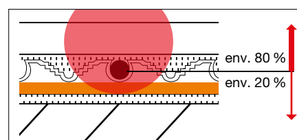
● Schlüter®-DITRA-HEAT-E-DUO avec barrière thermique
